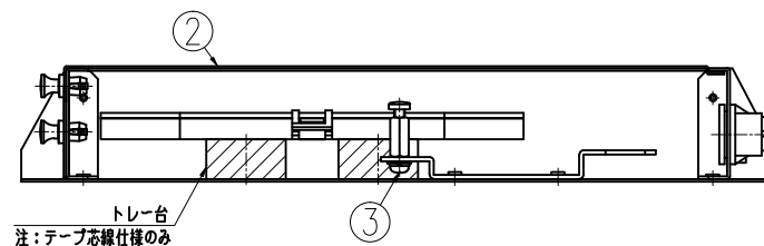
断面 AA
