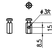
TMホルダ詳細図
