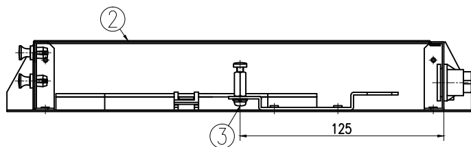
断面 AA
