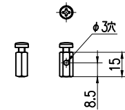
TMホルダ詳細図
