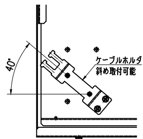
ケーブルクランプ斜め取付位置
