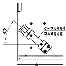
ケーブルクランプ斜め取付位置
