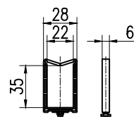
コードガイド寸法図
