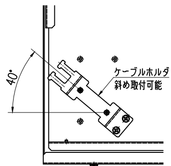
ケーブルクランプ斜め取付位置
