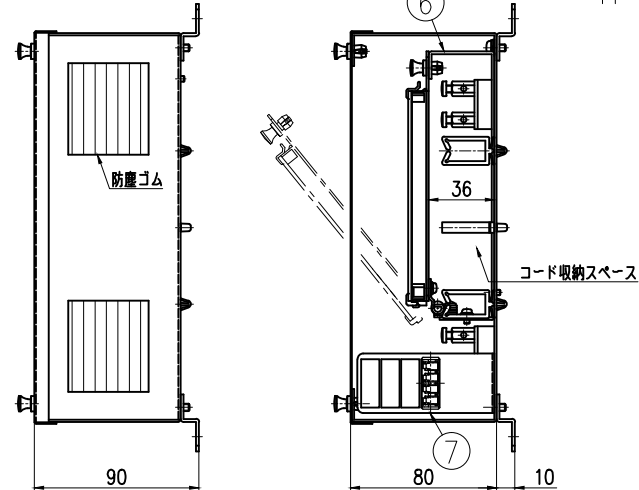
断面 BB
