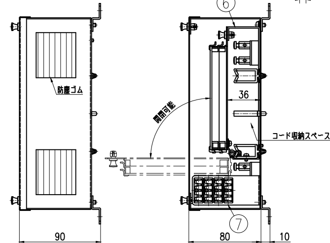
断面 BB
