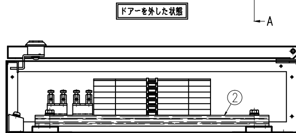
断面 BB
