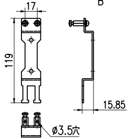
ケーブルホルダ詳細図
