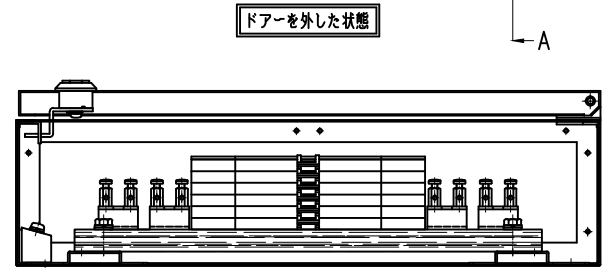
断面 BB
