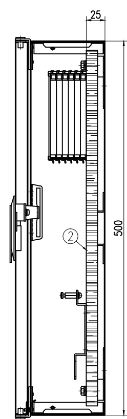
断面 AA
