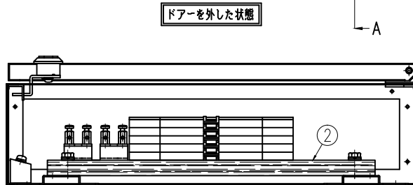
断面 BB
