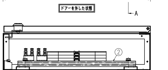
断面 BB
