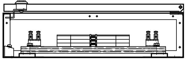
断面 BB
