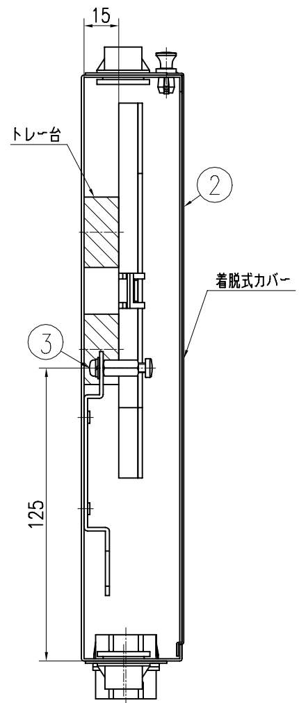
断面 AA
