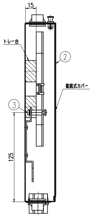
断面 AA
