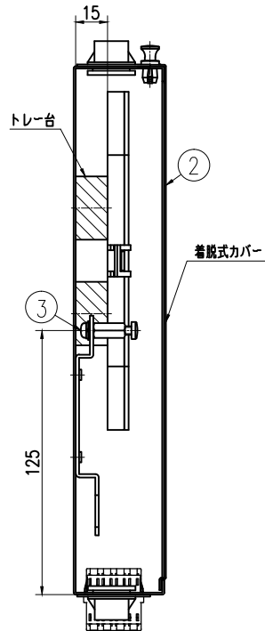
断面 AA
